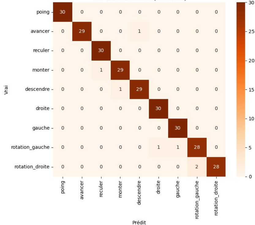
Matrice de confusion (validation)
