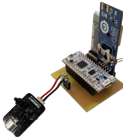
carte avec capteurs
